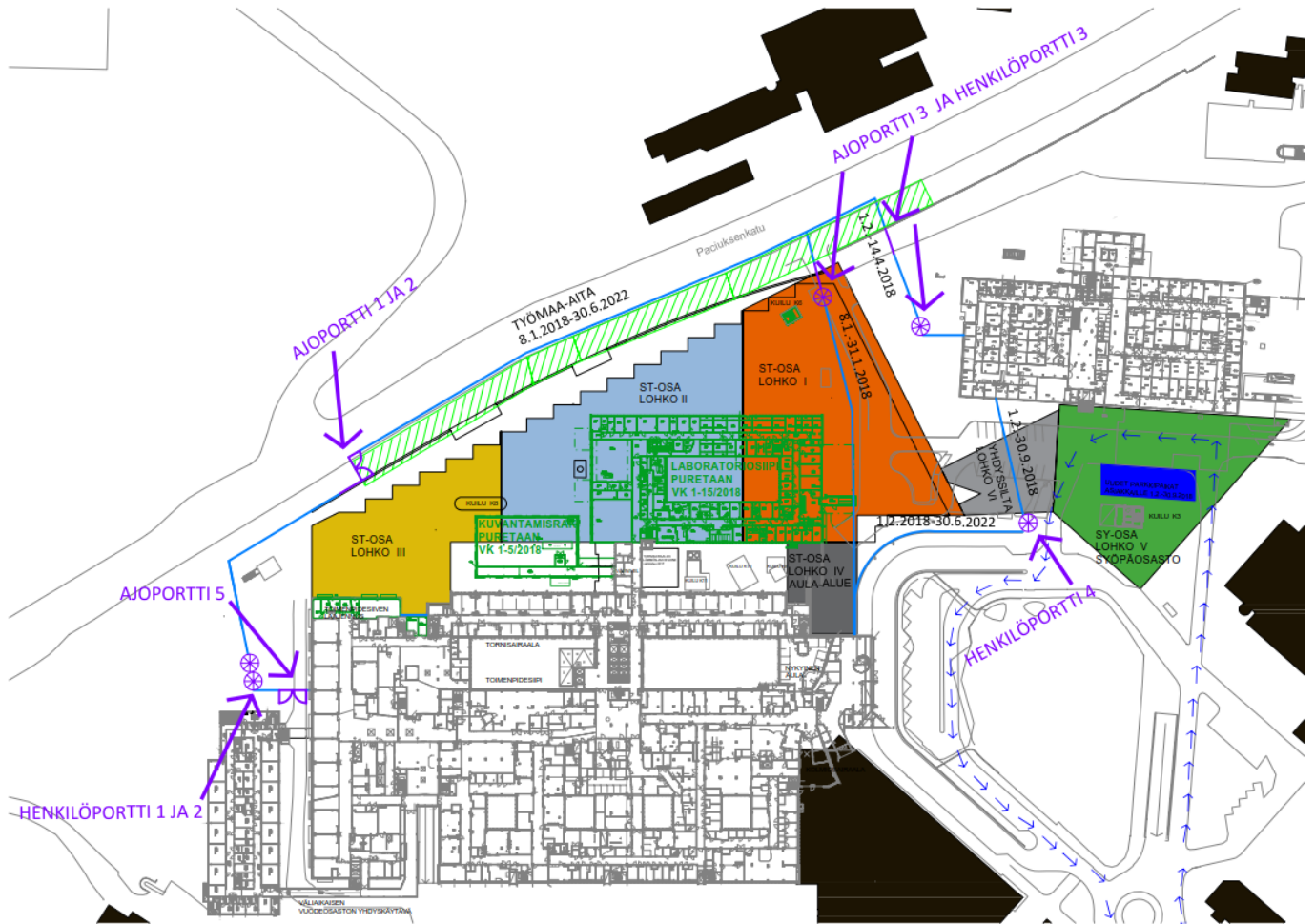
Kuva 3. Siltasairaalan työmaa-alue aitauksineen ja purettavine rakennuksineen vaiheiden 1 ja 2 aikana
